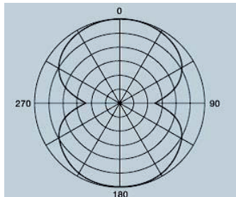
VHF波段方向图
